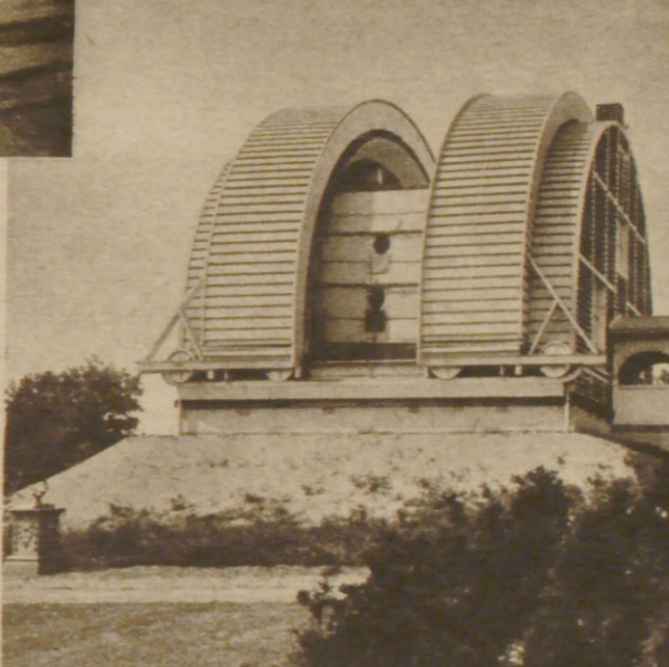
Gebäude des großen Meridiankreises. Das tonnenförmige Dach sorgt dafür, daß die unteren Luftschichten sich konzentrisch um die Drehachse des Instruments legen. So werden Störungen durch Lichtbrechung in den untersten Luftschichten vermieden
