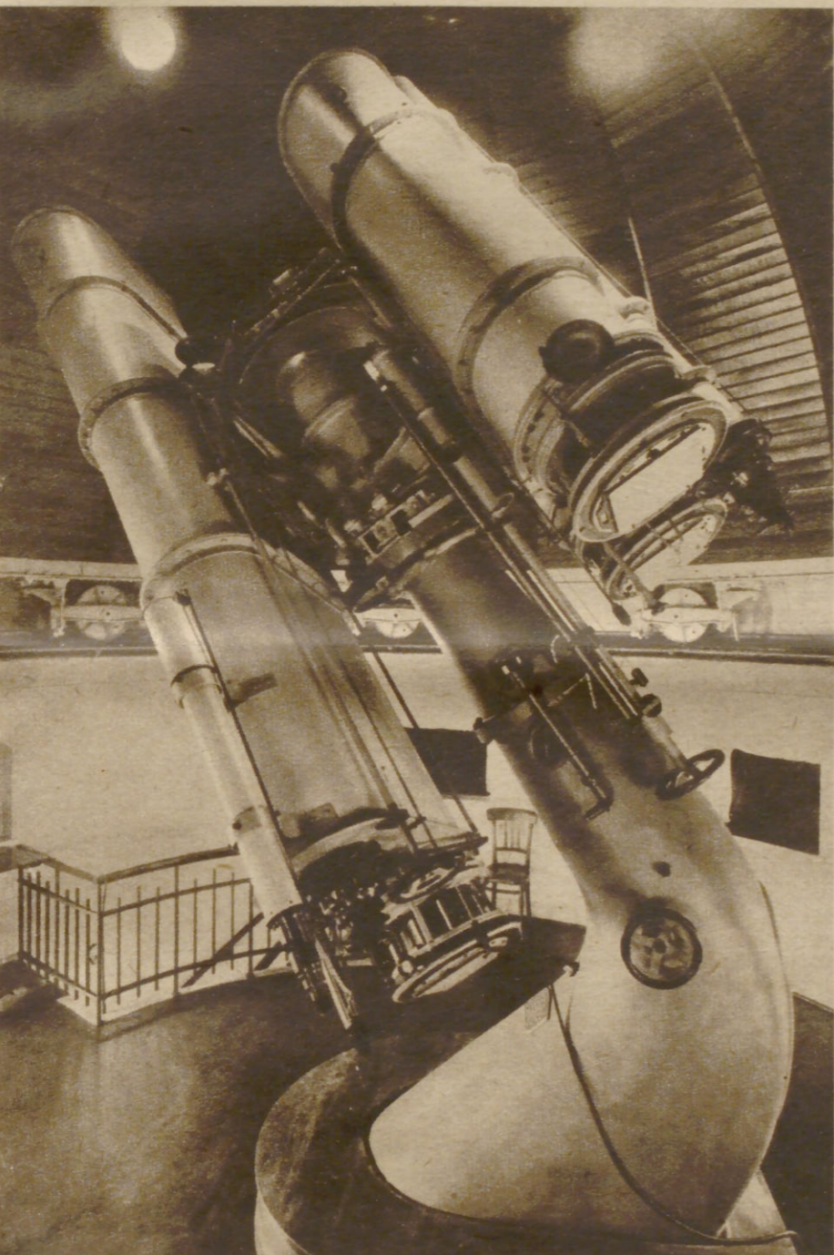
Der Lippert-Astragraph, mit dem die Bergedorfer Spektro-Durchmusterung durchgeführt wird. Zahlreiche kleine Planeten und einige Kometen wurden mit dem Instrument aufgefunden
