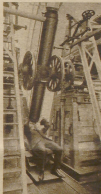
Der große Meridiankreis, das Hauptinstrument zur Zeitbestimmung und zur Messung von Sternörter
